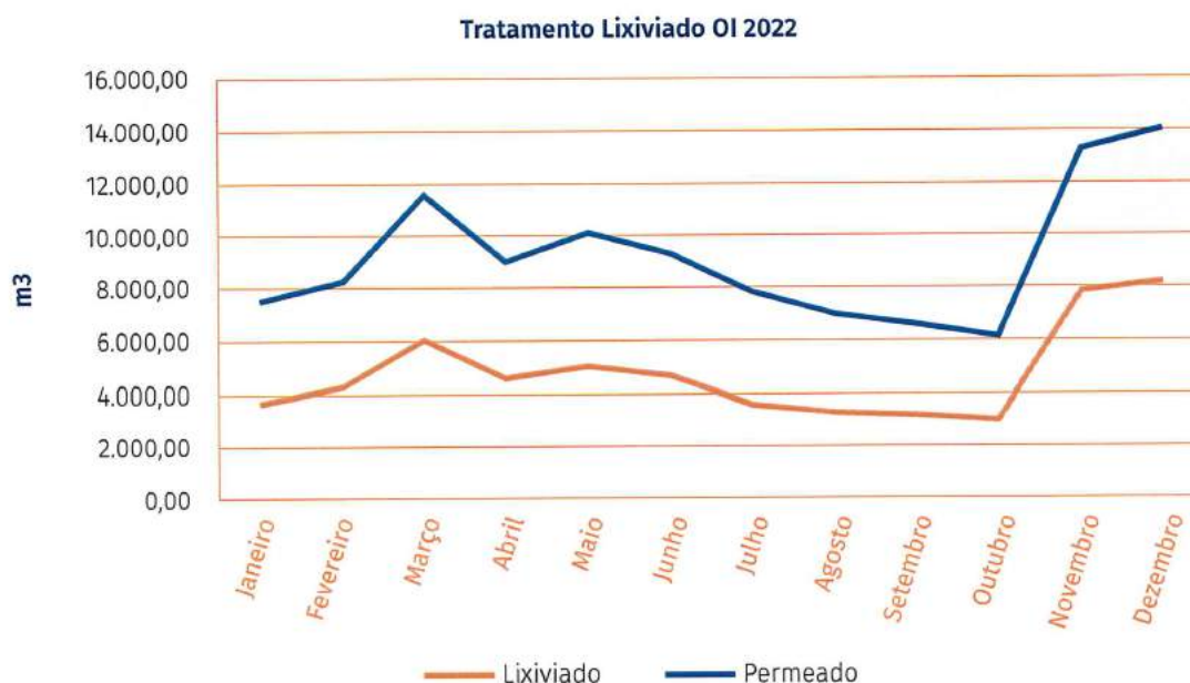
Figura 31 • Relação entre a quantidade de lixiviado e a quantidade de permeado
